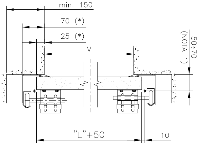
SEZ. A-A
